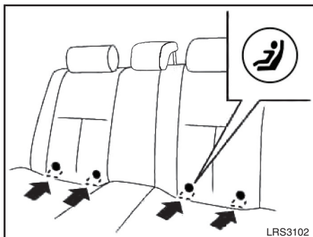
Localizações dos pontos de ancoragem inferiores do sistema ISOFIX
