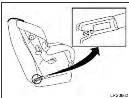
Fixação gancho rígido no sistema ISOFIX (se equipado)
