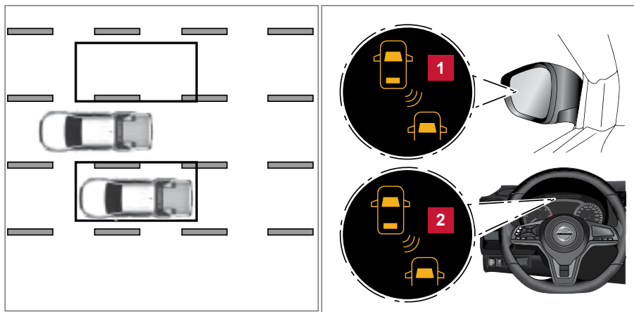
Zona de detecção
