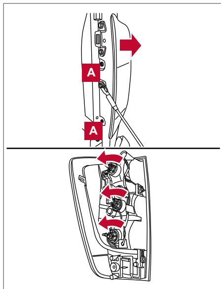
Luz combinada traseira
