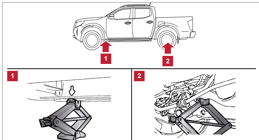
Pontos de levantamento
