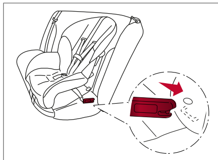
Fixação tipo gancho rígido voltado para frente - etapa 2
